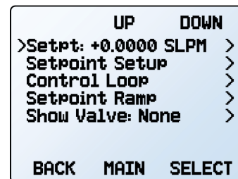
The control menu.
